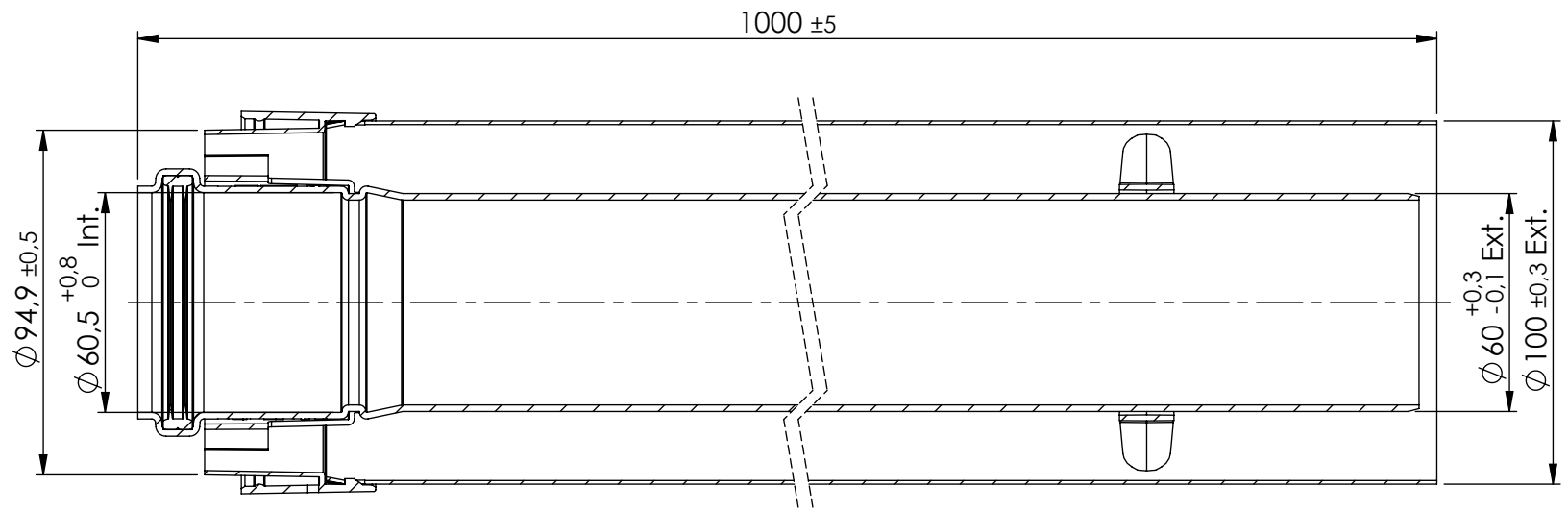
SECTION A-A
