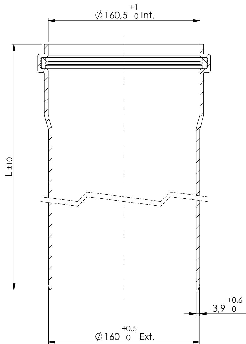
SECTION A-A
