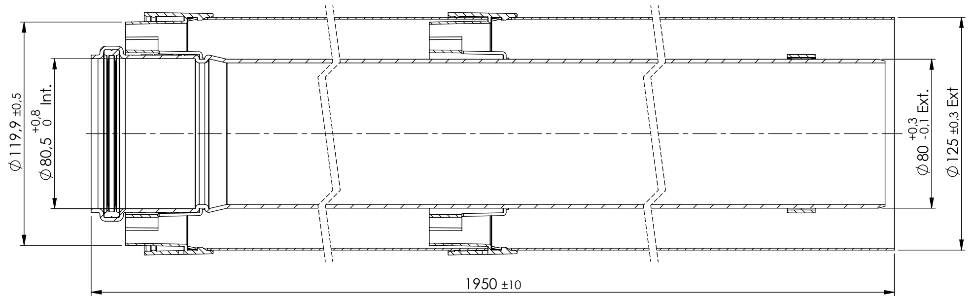
SECTION A-A
