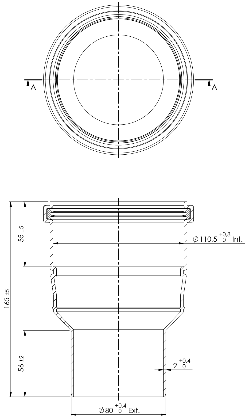
SECTION A-A
