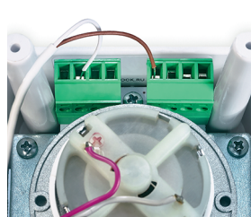
Фото 11. Подключение датчика к электроприводу
