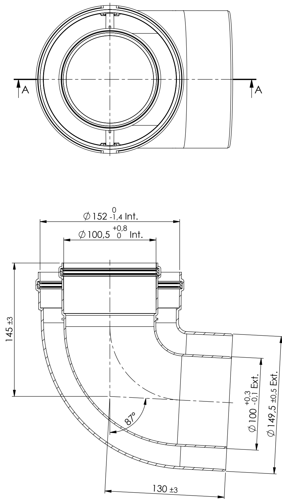
SECTION A-A
