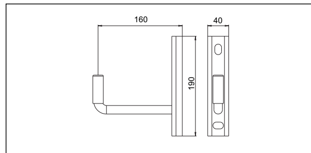
Натенный крепеж
