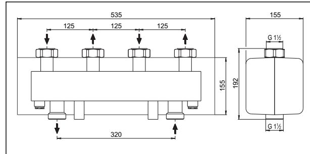
„HydroFixx“ Ду 25, на 2 отвода
