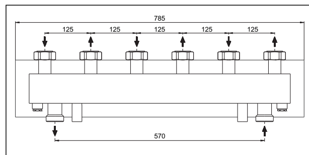
„HydroFixx“ Ду 25, на 3 отвода
