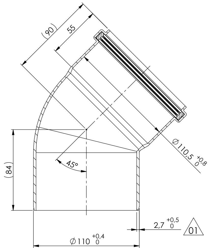
SECTION A-A
