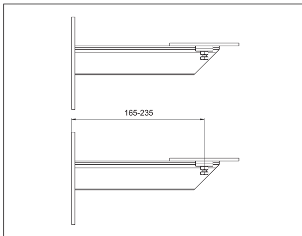
Размеры настенных консолей
