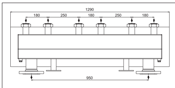
Размеры „HydroFixx“ DN40/50, на 3 контура
