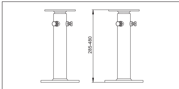
Размеры напольных консолей
