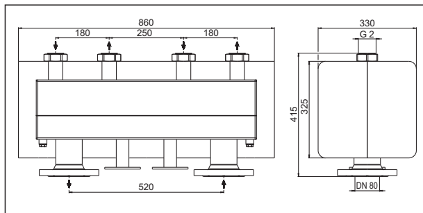
Размеры „HydroFixx“ DN 40/50, на 2 контура
