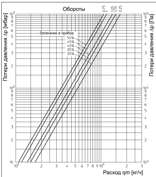
ZBU-, CEW-присоединительные узлы для однотрубных систем
