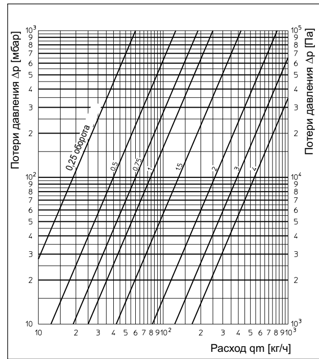
ZV-присоединительные узлы Артикул №: 101 62 41/42 101 62 91/92
