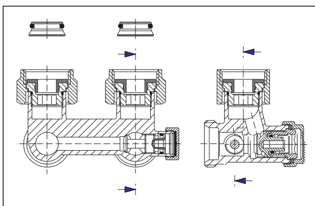
ZBU-угловой присоединительный узел с функцией слива, заполнения и преднастройки, артикул №: 101 59 44
