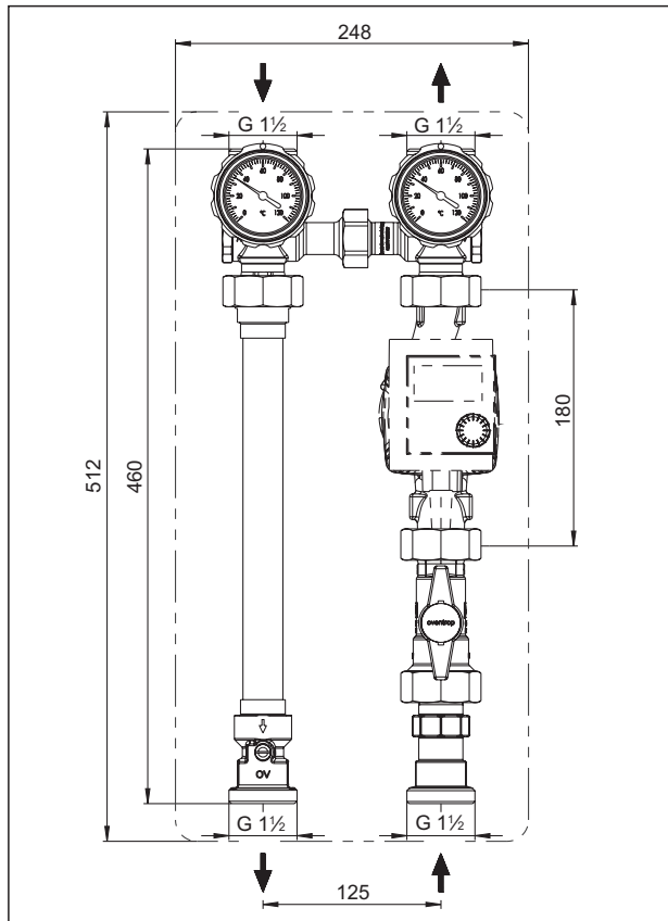
„Regumat S-180“ Ду 25 с шаровым краном перед насосом
