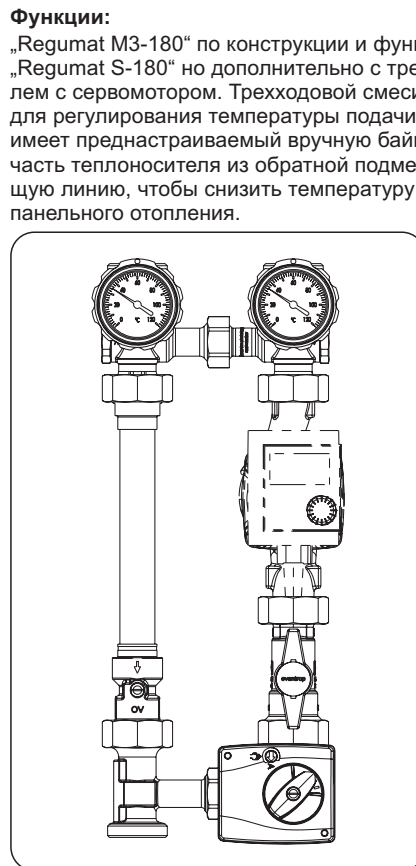
„Regumat M3-180“
